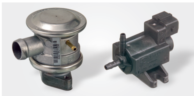
Válvula de retenção desconectável regulada por vácuo (a partir de aprox. 1995) e válvula de comutação
